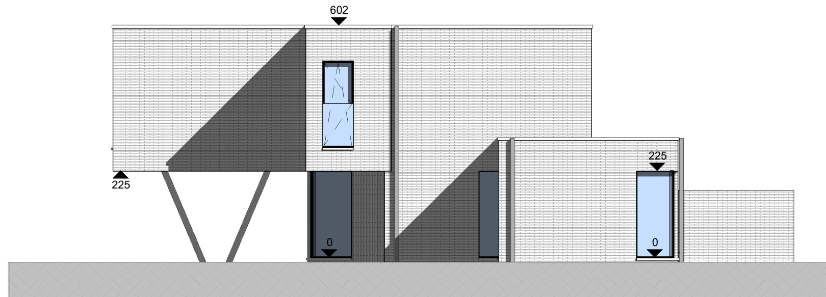
③ Rechter zijgevel woning 9 1 : 100
