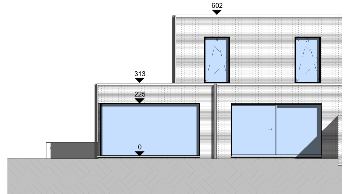
② Achtergevel woning 9 1 : 100
